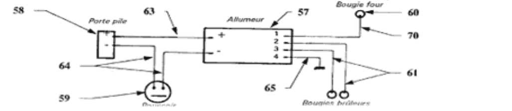
SCHEMA DU CABLAGE POUR ALLUMEUR 1,5 Volt
