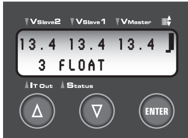
SBC 700 NRG FR - SBC 1100 NRG FR
