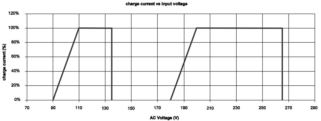
Abbildung 15: Ladestrom im Vergleich zu Eingangsspannung
