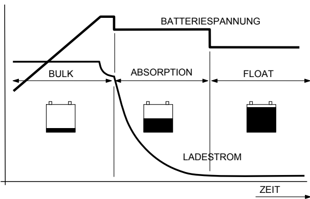
Abbildung 4: Dreistufen-Plus-Ladesystem
