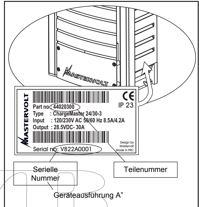
Abbildung 1: Typenschild
