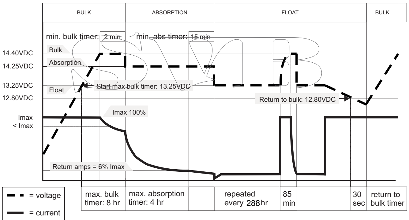
Abbildung 16: Ladekennlinie der Dreistufen-Plus-Lademethode (@ 25°C / 77°F)
