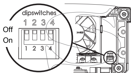
Abbildung 7: DIP Schalter
