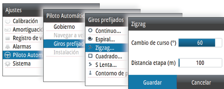
Ajustes de giros prefijados, AP44
