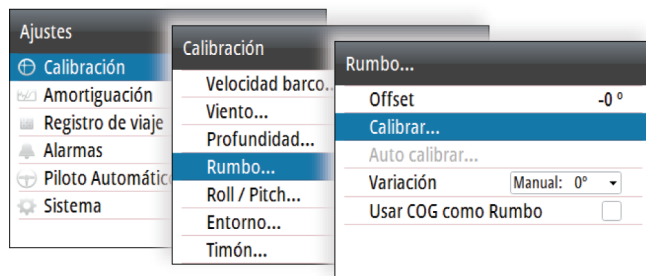
Opción Calibración, AP44
