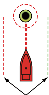
XTE lines
