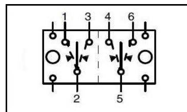
Anschlussbelegung Tast-Kontakte
