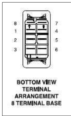
Kontaktbelegung, Sicht auf Tasterunterseite
