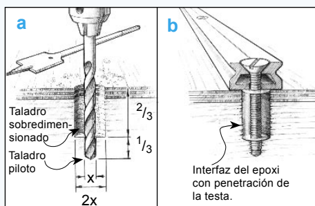
Figura 16 Practique taladros sobredimensionados con el fin de aumentar la zona expuesta del sustrato y la cantidad de epoxi alrededor de la fijación.
