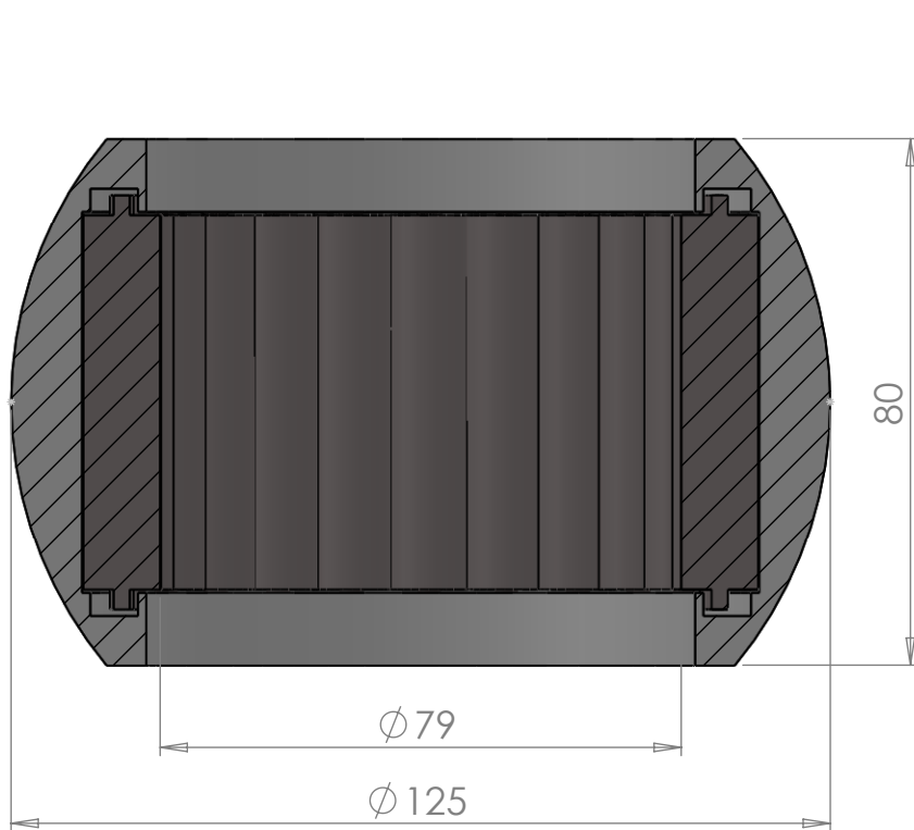
SECTION A-A SCALE 1 : 1.25
